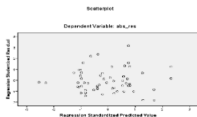
Gambar 2 Grafik Scatterplot
