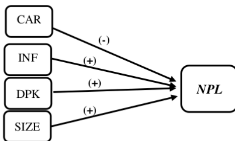
Gambar 1. Kerangka Pemikiran
