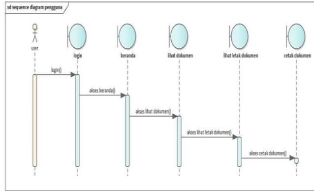
Gambar 6. Sequence Diagram pengguna
