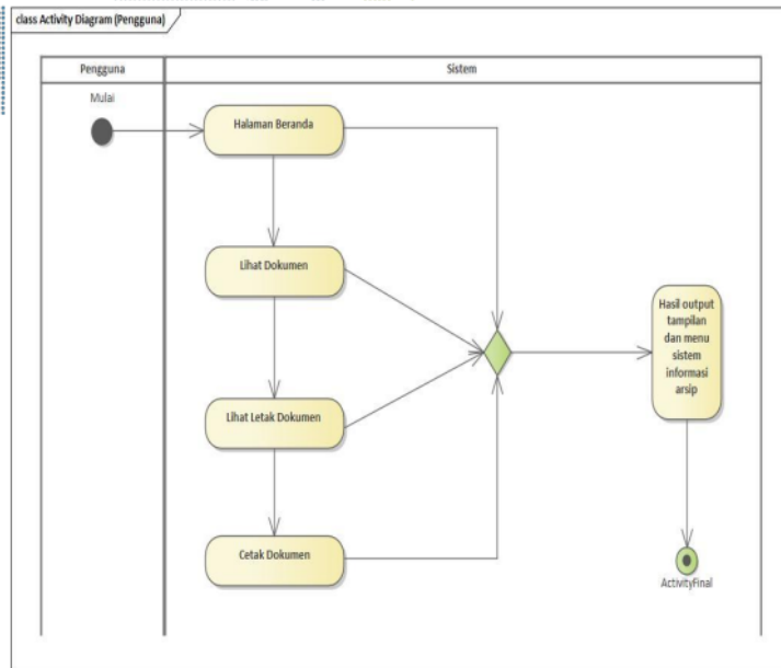
Gambar 4. Activity Diagram (pengguna)
