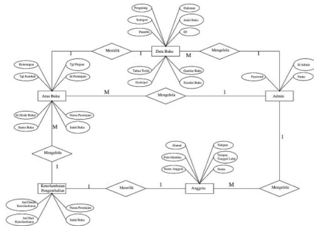
Gambar 4. ERD (Entity Relationship Diagram) Desain Sistem Informasi Perpustakaan Universitas Stikubank Semarang Berbasis Web
