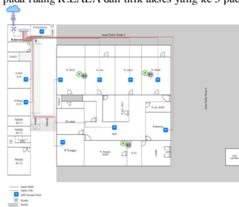
Gambar 4.2 Lokasi titik akses
