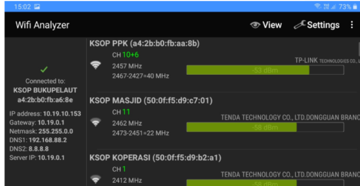
Gambar 4.5 Detail nilai dBm titik akses
