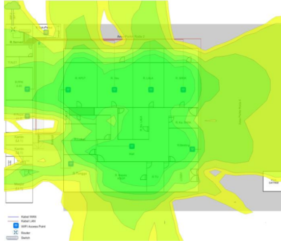
Gambar 4.3 Coverage area dengan Ekahau Heatmapper
