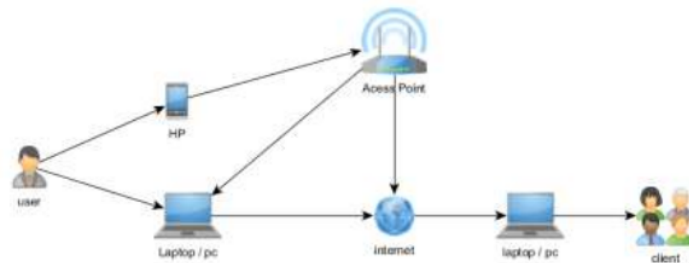
Gambar 7. Skenario Pengujian
