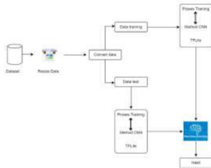
Gambar 3. Diagram Deteksi Penyakit Kulit Wajah
