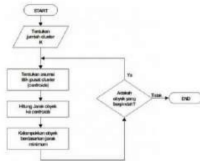
Gambar 1 Algoritma K-means
