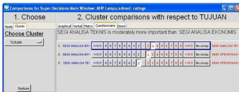
Gambar 2. Perbandingan Kriteria dengan Tujuan
