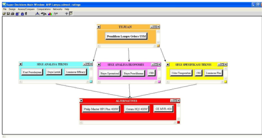
Gambar 1. Susunan Hirarki Permasalahan
