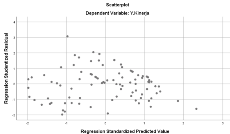
Gambar 2. Uji Heterokedastitas
