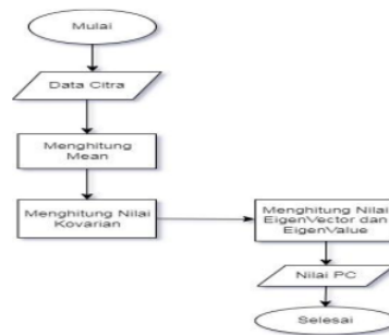
Gambar 4. Flowchart PCA
