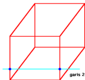
Gambar 12 Garis 2 pada ruang dimensi tiga
