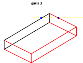
Gambar 13. Garis 3 pada ruang dimensi tiga
