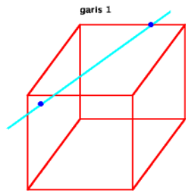
Gambar 11. Garis 1 pada ruang dimensi tiga
