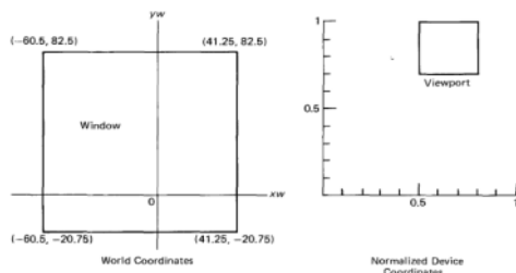
Gambar 2. Jendela dan sistem koordinat (Hearn dan Baker, 1986)
