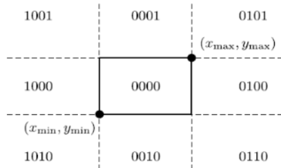
Gambar 6 Kode 4 bit algoritma Cohen-Sutherland (klawonn, 2012)
