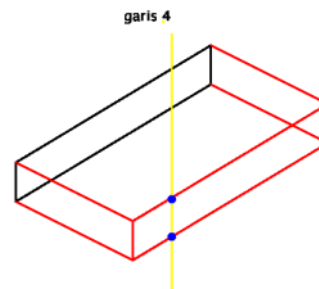
Gambar 14 Garis 4 pada ruang dimensi tiga
