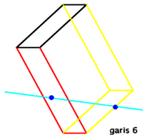
Gambar 16 Garis 6 pada ruang dimensi tiga
