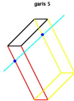
Gambar 15. Garis 5 pada ruang dimensi tiga
