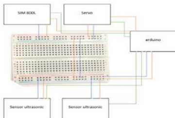
Gambar 2. Gambaran rangkaian
