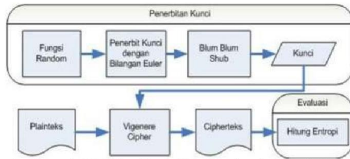
Gambar 3 Desain Modifikasi Penerbitan Kunci pada Extended Vigenere
