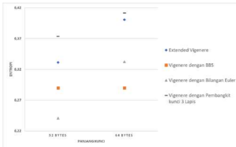
Gambar 5 Perbandingan nilai entropi Extended Vigenere menggunakan pembangkit kunci berlapis dengan penelitian sebelumnya
