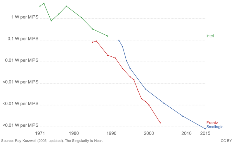
Gambar 18.2: Efisiensi Kinerja Processor
