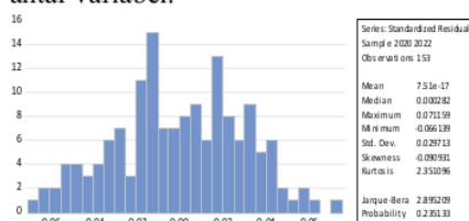
Gambar 2. Uji Normalitas
