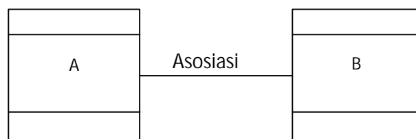
Gambar 3.11 Relasi Asosiasi
