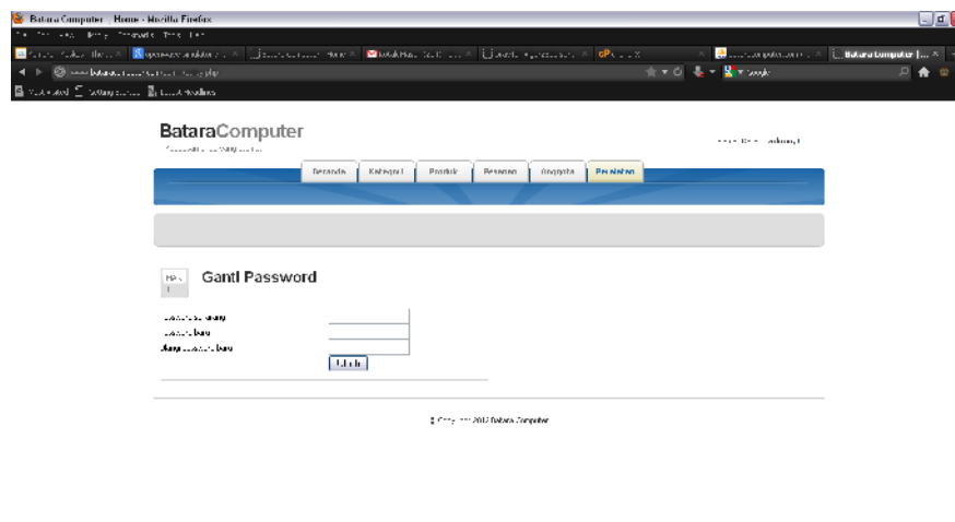
Gambar 5.39 Halaman Peralatan
