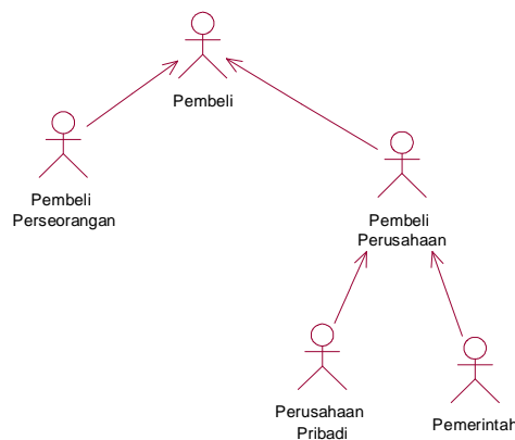
Gambar 3.8 Contoh Relasi Generalisasi
