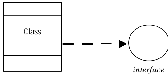
Gambar 3.14 Realisasi
