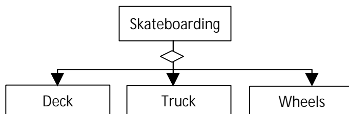
Gambar 3.13 Agregasi
