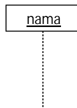
Gambar 3.16 Objek
