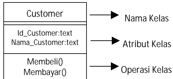
Gambar 3.10 Notasi Atribut
