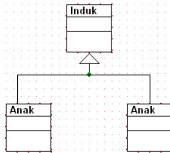
Gambar 3.15 Notasi Generalisasi
