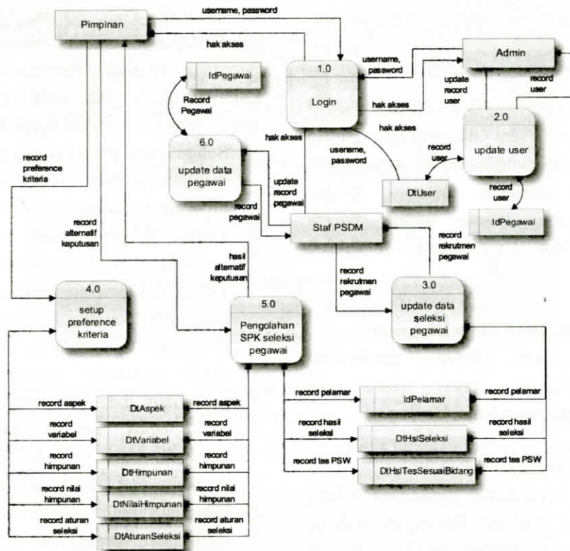
Gambar 12. DFD level 1 Sistem Pengambilan Keputusan Seleksi Sesuai bidang
