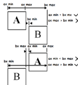
Gambar 3. bound tidak bertabrakan
