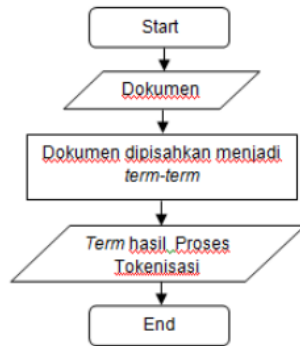
Gambar 8. Flowchart Proses Tokenisasi
