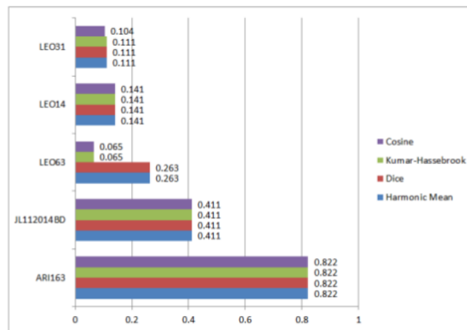
Gambar 4. Bobot Dokumen semua metode pada keyword Wong seneng ngalah
