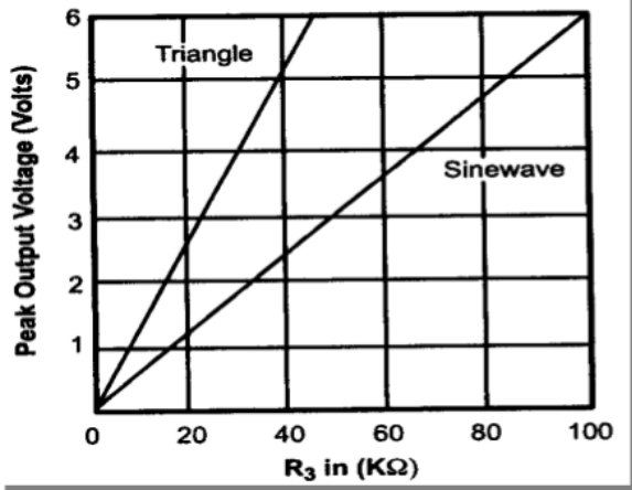
Gambar 4. Grafik Amplitudo – Harga Resistor R3
