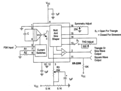
Gambar 3. Rangkaian Pembangkit Pulsa
