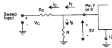
Gambar 11. Rangkaian Pengatur Frekuensi
