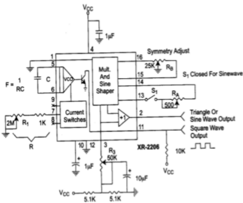
Gambar 8. Rangkaian Penghasil Sinyal Sinusoidal dengan Distorsi Rendah
