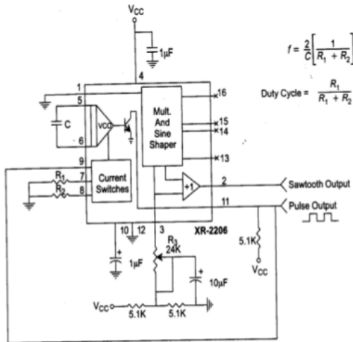
Gambar 10. Rangkaian Generator Pulsa
