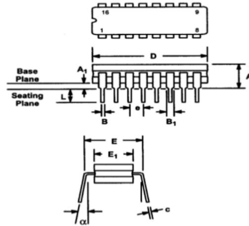
Gambar 2. IC XR-2206
