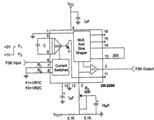
Gambar 9. Generator FSK Sinusoidal
