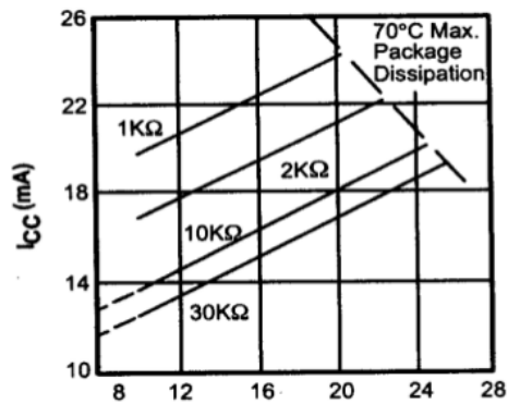
Gambar 5. Grafik Arus dan Tegangan Catu Daya, Pewaktu dan Resistor
