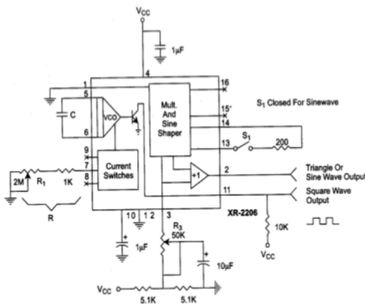
Gambar 7. Rangkaian Penghasil Sinyal Sinusoidal
