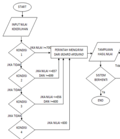
Gambar 4. Flowchart Sistem Rancang Bangun
