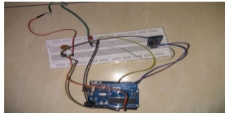
Gambar 7. Rancang Bangun pada Arduino UNO
