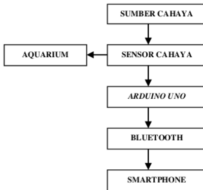
Gambar 3. Diagram Blok Rancang Bangun Turbidimeter
