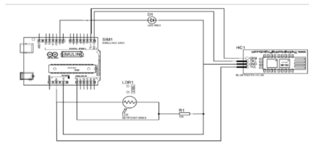
Gambar 2. Skema Rangkaian Sistem
