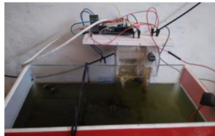
Gambar 9. Implementasi Rancang Bangun Pada Aquarium
