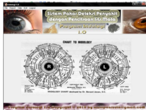
Gambar 14 Form Utama
