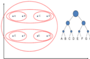
Gambar 1. Contoh algoritma HAC
