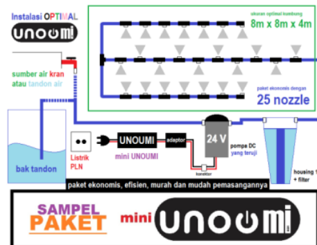
Gambar 4. Sampel Standar Instalasi mini UNOUMI set lengkap
