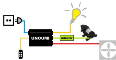
Gambar 1. Rangkaian Standar Uji Implementasi Sistem UNOUMI
