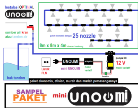
Gambar 5. Sampel Standar Instalasi alternatif mini UNOUMI
