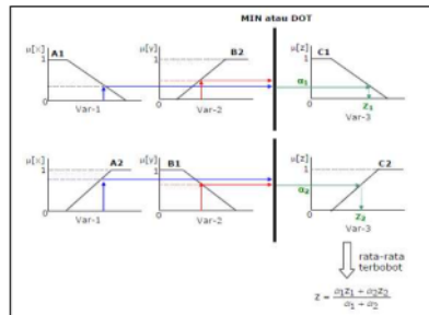
Gambar 7 komposisi fuzzy Sugeno
