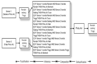
Gambar 3. Variabel, himpunan dan aturan fuzzy dalam FIS
