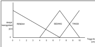
Gambar 4 Fungsi keanggotaan sensor 1
