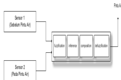
Gambar 2. Inference Proses Sistem Informasi Ketinggian Air dan Pintu Air
