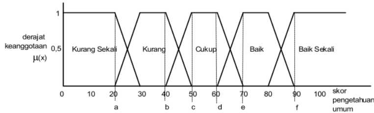
Gambar 20. fungsi keanggotaan pengetahuan umum
