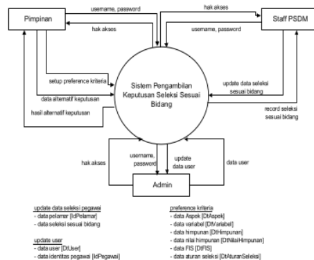
Gambar 11. Diagram Konteks Sistem Pengambilan Keputusan
