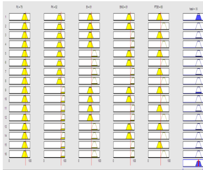
Gambar 27. Hasil proses komposisi untuk seleksi sesuai bidang
