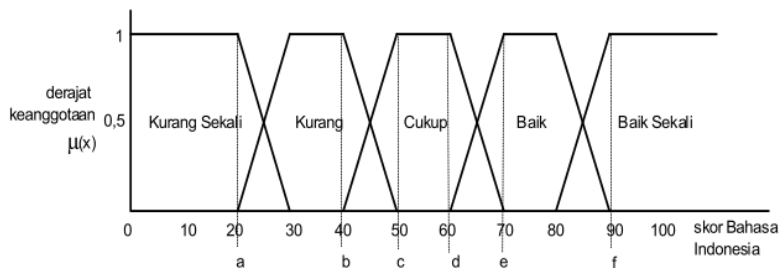
Gambar 6. Fungsi keanggotaan Bahasa Indonesia
