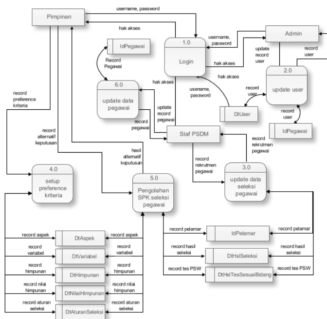
Gambar 12. DFD level 1 Sistem Pengambilan Keputusan Sesuai bidang
