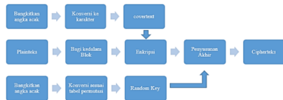
Gambar. 1. Usulan Modifikasi Model Enkripsi ECR.
