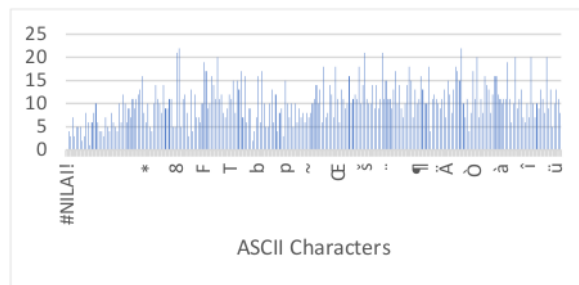
Gambar. 3. Histogram karakter ciphertexts hasil ECR modifikasi
