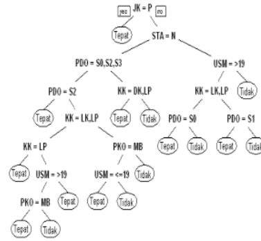
Gambar 3. Pohon keputusan dengan ujung berupa nama kelas
