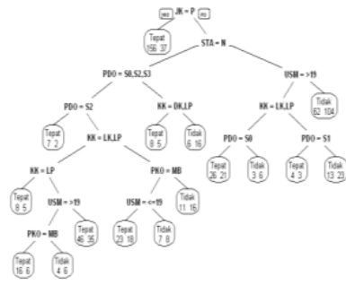
Gambar 4. Pohon keputusan dengan Jumlah data
