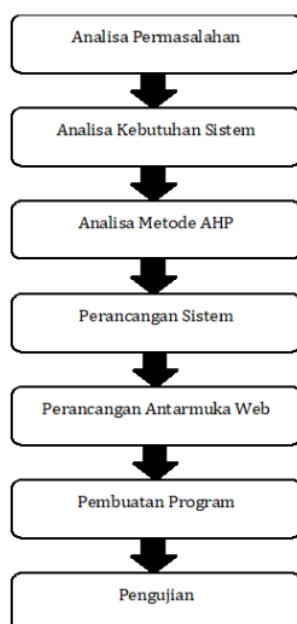
Gambar 1. Tahapan Penelitian.
