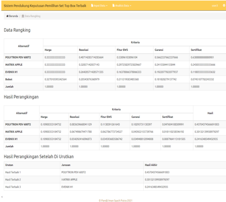
Gambar 7. Hasil Perangkingan.
