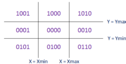
Gambar 3. Kode area Cohen-Sutherland dimensi dua.
