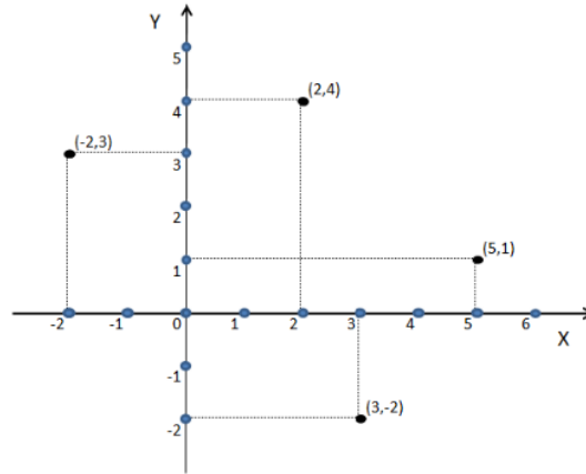
Gambar 1. Koordinat Kartesius pada bidang dimensi dua.
