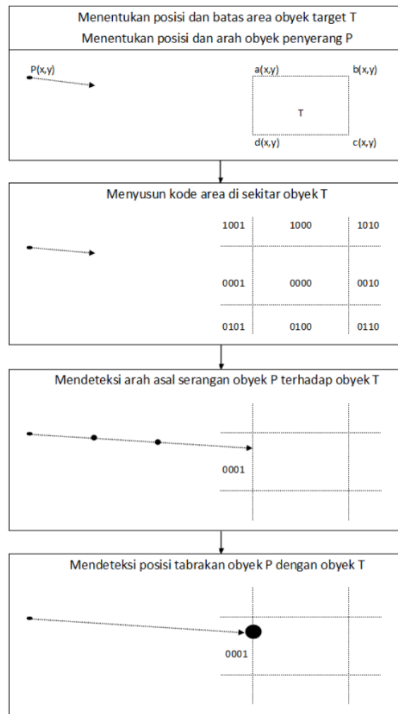
Gambar 6. Blok diagram langkah penelitian.
