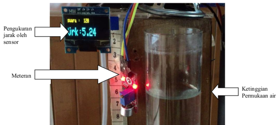
Gambar 7. Hasil pengamatan ketinggian air
