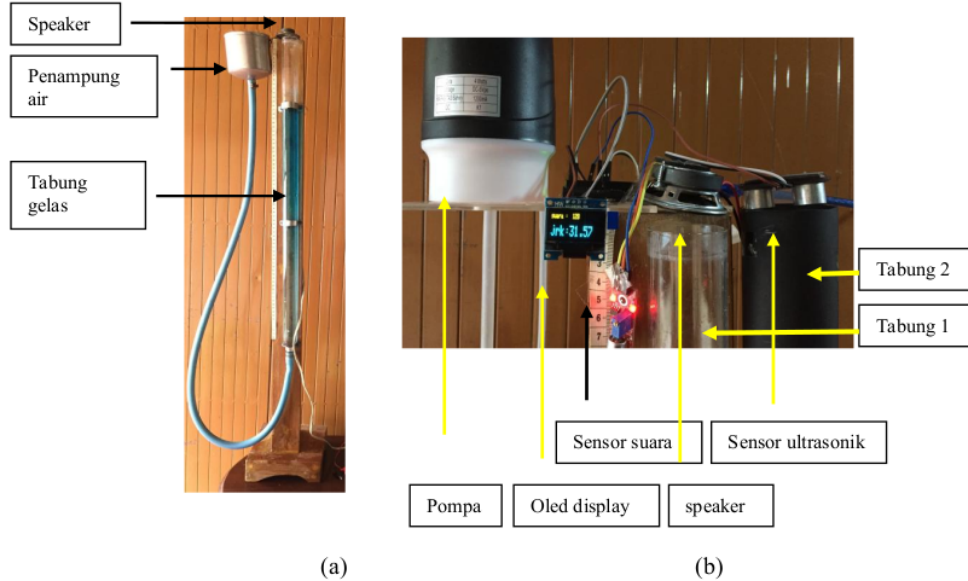
Gambar 6. Tabung Resonansi tanpa sensor(a), tabung resonansi dengan sensor dan oled display(b)
