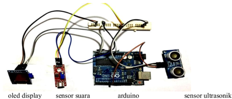
Gambar 4. Tata letak arduino, modul sensor dan oled display
