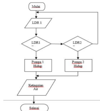
Gambar 5. Diagram Alir Kendali Sensor dan Pompa
