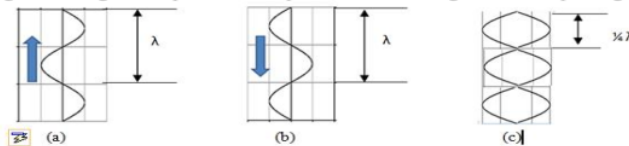
Gambar 1. Gelombang masuk tabung(a), gelombang pantul (b), gelombang interferensi(c)
