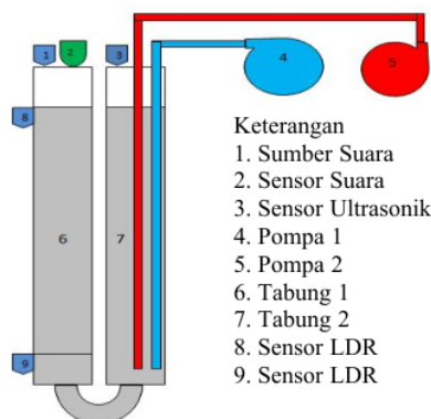
Gambar 4. Tata Letak tabung dan Komponen Elektronik
