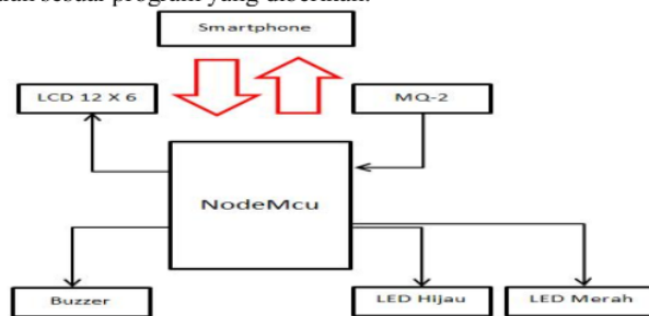
Gambar 1. Diagram blok, konsep rancangan
