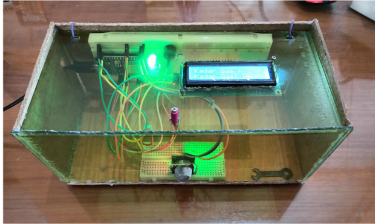
Gambar 7. alat keseluruhan
