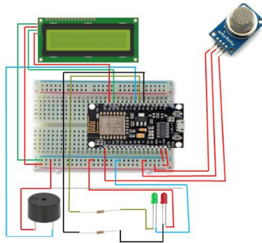
Gambar 6. Konsep rangkaian keseluruhan
