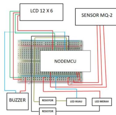
Gambar 4. Simulasi rangkaian alat
