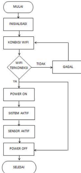
Gambar 2. Flowchart aplikasi
