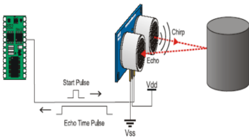
Gambar 5. Cara kerja sensor ultrasonik
