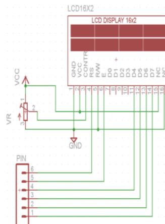
Gambar 7. Konfigurasi LCD
