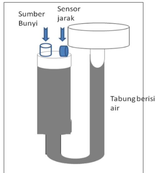
Gambar 8. Tata letak sensor dan sumber bunyi
