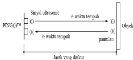
Gambar 6. Perhitungan jarak sensor dan objek
