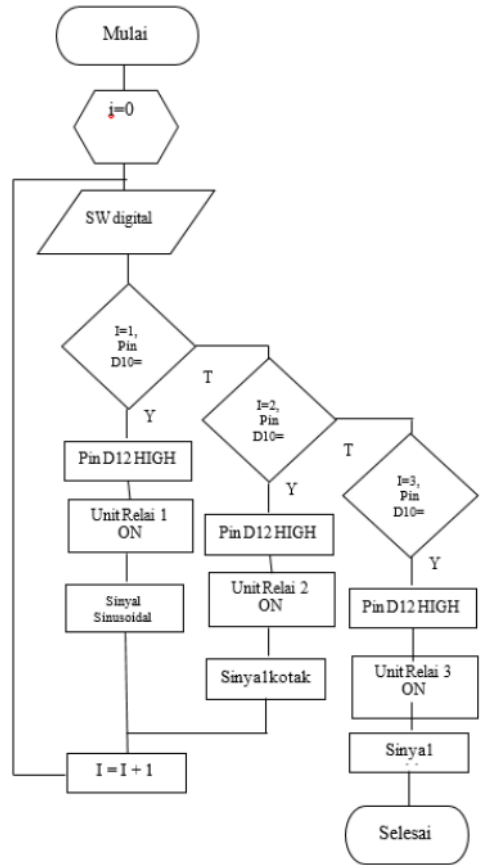
Gambar 8. Flowchart Pengendali sinyal
