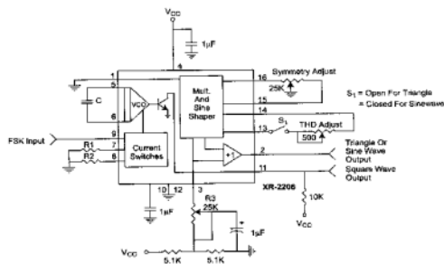
Gambar 3. Rangkaian IC XR-2206
