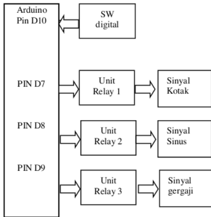
Gambar 7. Alur kerja pengendali sinyal
