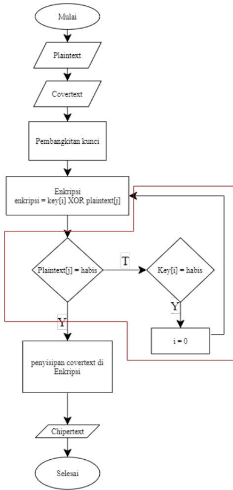
Gambar 2. Enkripsi PDAC teknik pengulangan kunci
