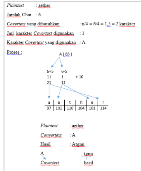
Gambar 1. Enkripsi PDAC dengan covertext kurang dari n/4
