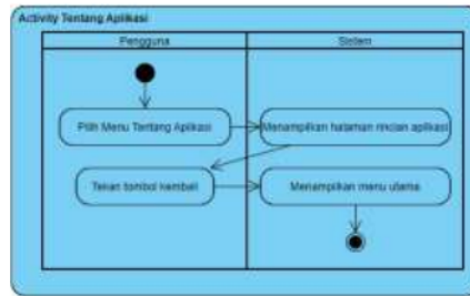
Gambar 6 Activity Diagram Tentang Aplikasi
