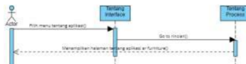
Gambar 9 Sequence Diagram Tentang Aplikasi
