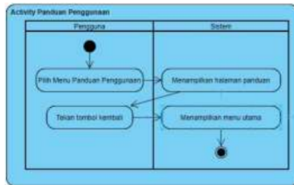
Gambar 5 Activity Diagram Panduan Penggunaan
