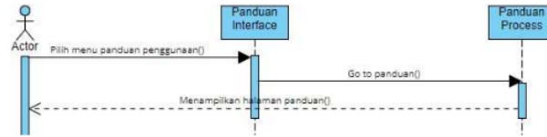
Gambar 8 Sequence Diagram Panduan Penggunaan
