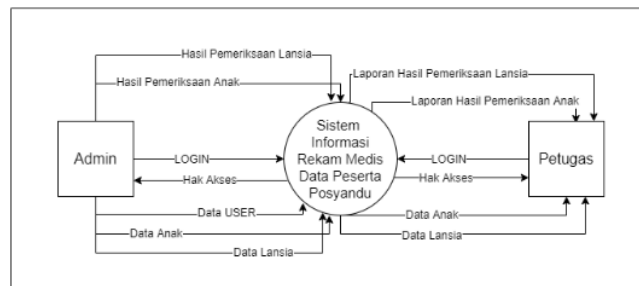
Gambar 2. Diagram Konteks
