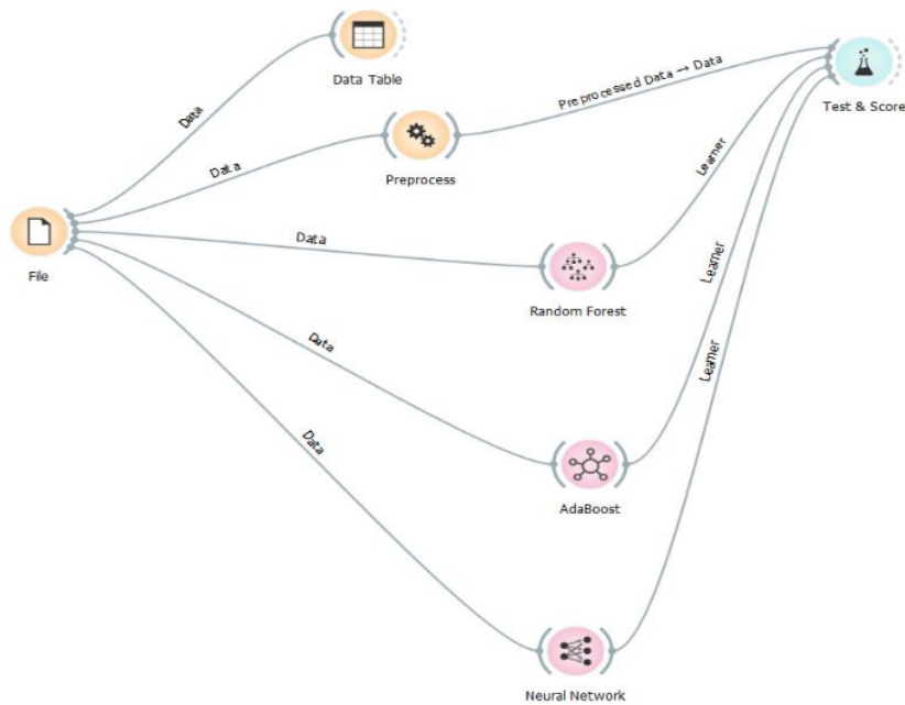
Gambar 4: Desain Aplikasi Orange
