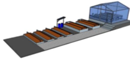
Gambar 4 : Grand Design Tehnologi Terapan Kebun Nandur Sedekah
