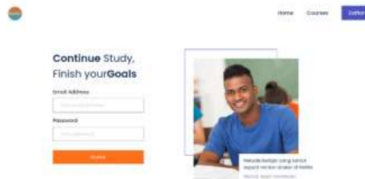
Gambar 12 Halaman Login
