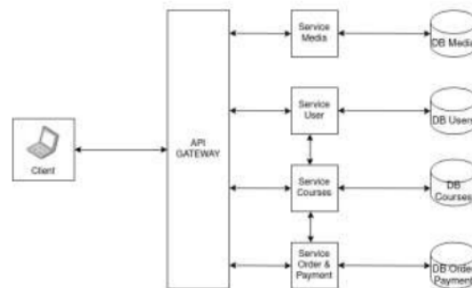
Gambar 3 Rancangan Arsitektur Microservices
